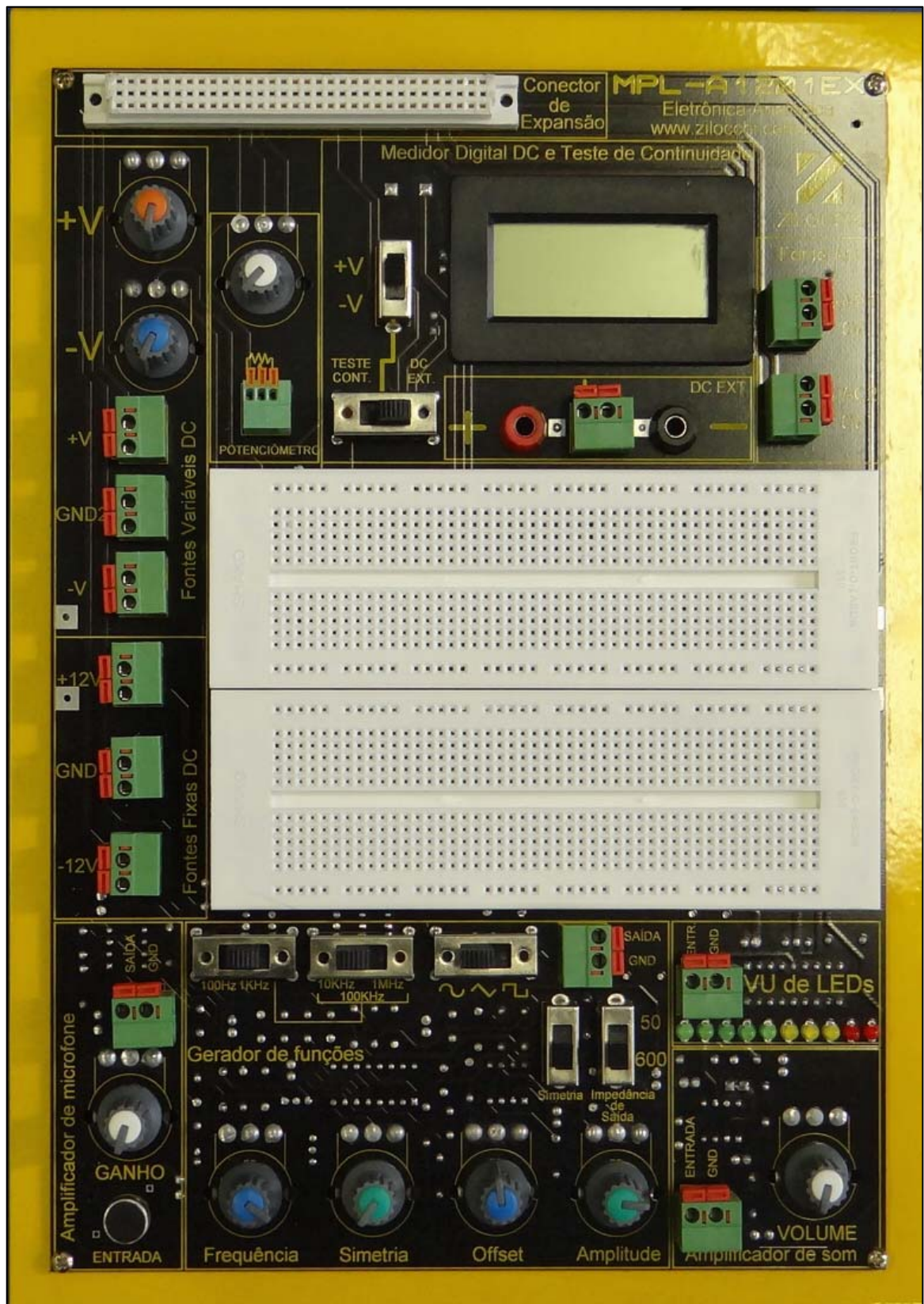
FIGURA 2 - Módulo Educacional de Treinamento para Eletrônica Analógica, modelo MPL-A1201EX, marca ZILOCCHI
